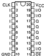
THCTPAL16R6-M . . . J PACKAGE THCTPAL16R6-C . . . J OR N PACKAGE (TOP VIEW)
