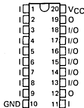
THCTPAL16R4-M . . . J PACKAGE THCTPAL16R4-C . . . J OR N PACKAGE (TOP VIEW)
